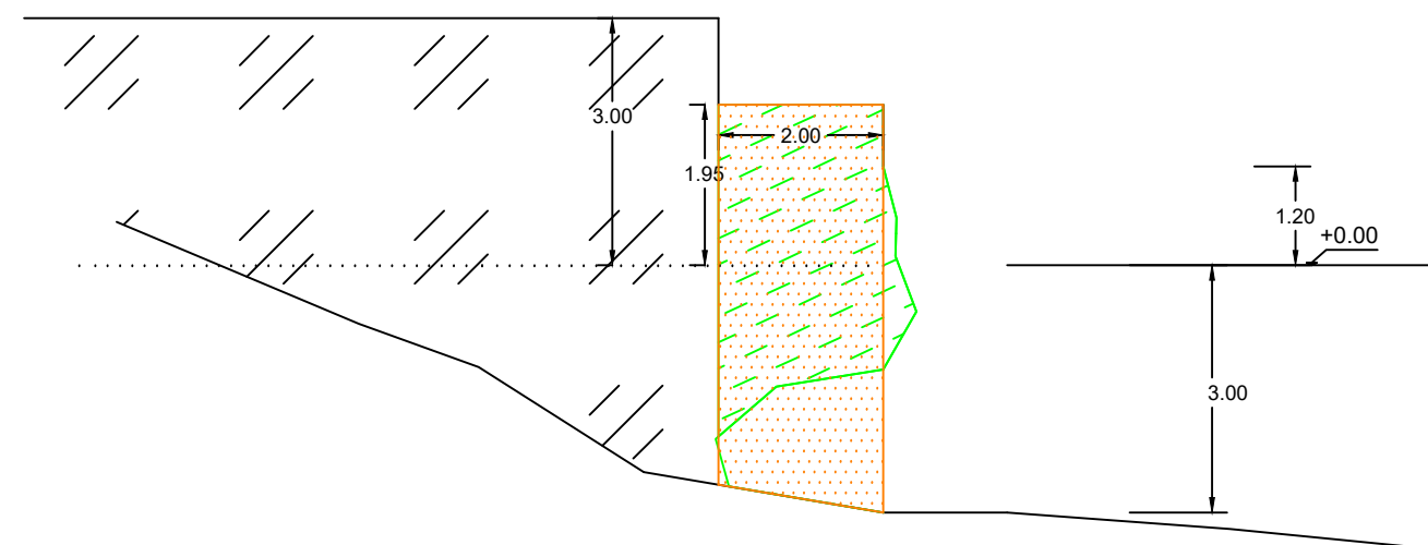
Τομή στη θέση Γ - Ακρομώλιο
