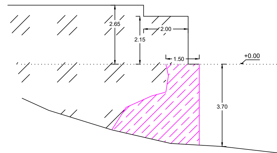
Τομή στη θέση Γ - Ακρομώλιο
