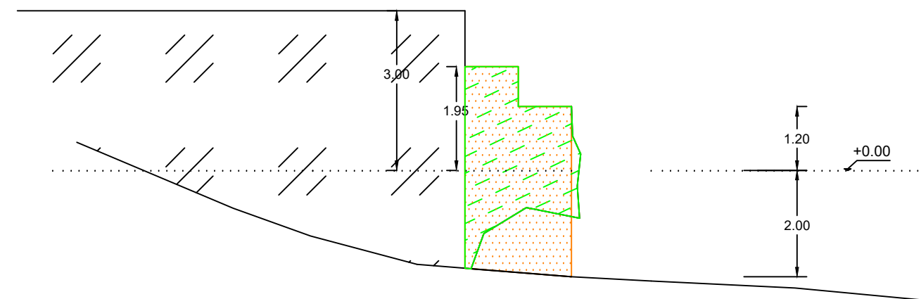
Τομή στο κρηπιδώμα ΑΒ στη θέση Β
